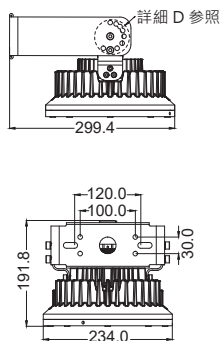
壁取付 90° (W90-2)
