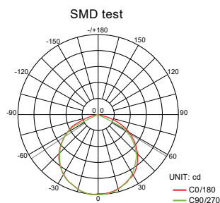
極座標配光曲線
